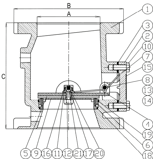
Рис. 2. Конструкция клапана
