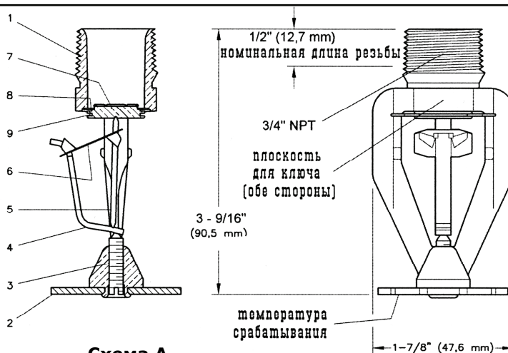
Схема А Быстродействующий спринклерный ороситель для раннего подавления огня ESFR-17 с плоской розеткой
