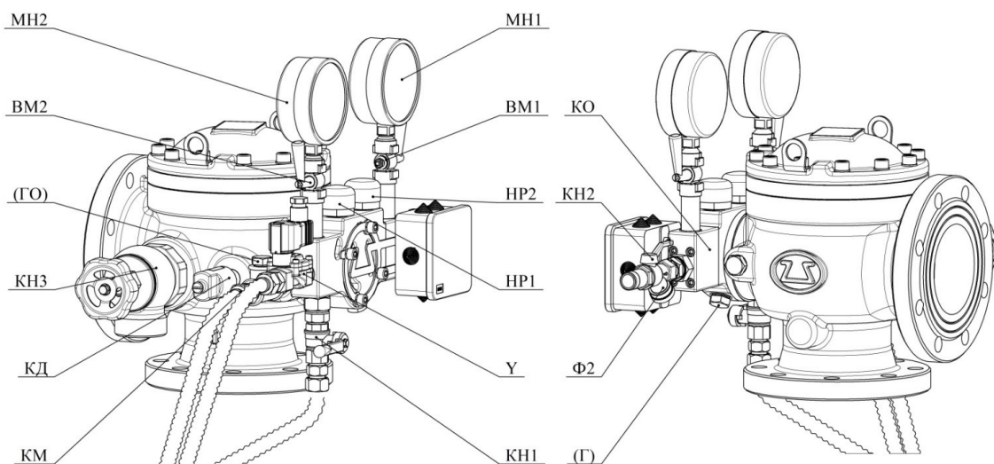
Рисунок 3 - Узел управления дренчерный с комбинированным приводом
