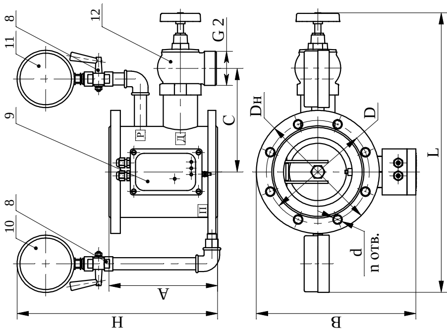
Рисунок 1 - Узел управления sprinklerный водозаполненный с сигнализатором потока жидкости
