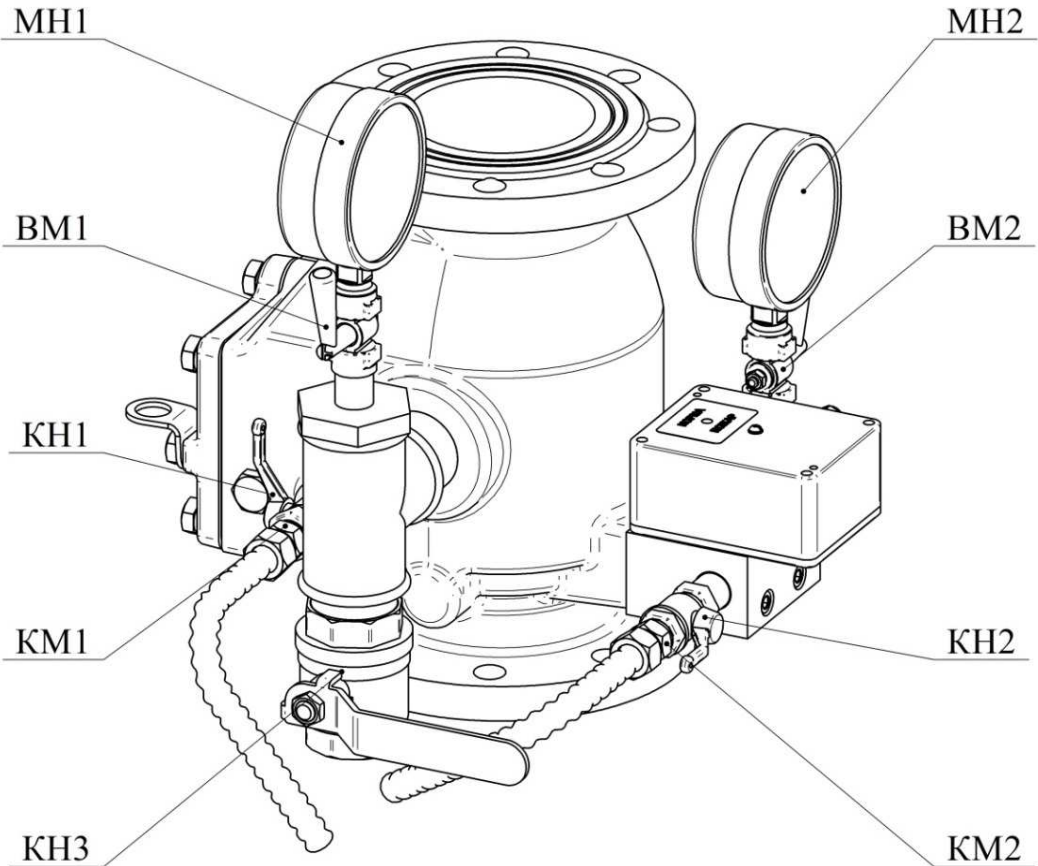
Рисунок 4 - Узел управления спринклерный водозаполненный DN100, 150 с устройством задержки
