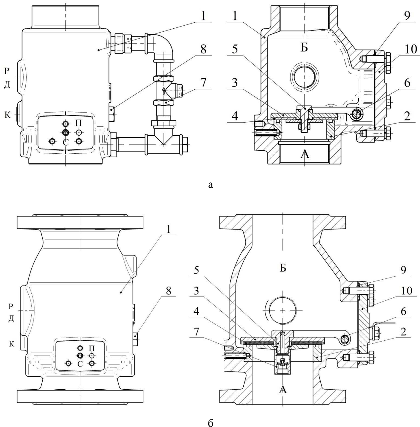
Рисунок 1 - Клапан сигнальный спринклерный «Баге плюс»
