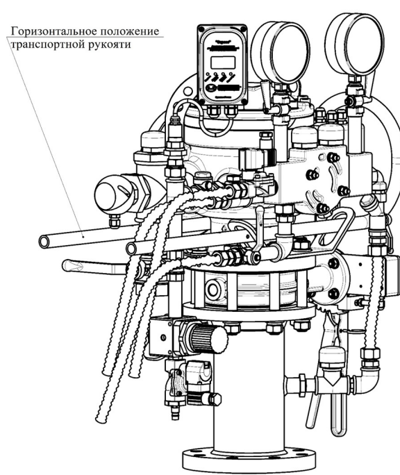
Рисунок 3 — Горизонтальное положение транспортной рукоятки
