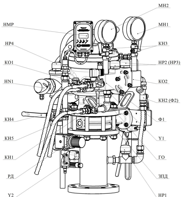
Рисунок 2 — Общий вид УУ «Спринт-100 (150)»
